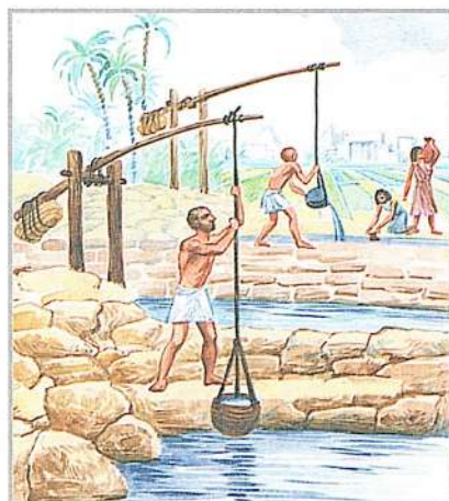
Шадуф. Современный рисунок
